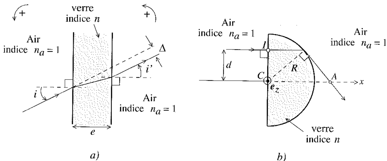
FIG. 1 - (a) Lames à faces parallèles et (b) lentille hémicylindrique d'axe de révolution Ce_z .
