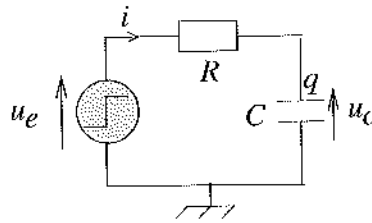
FIG. 3 Circuit RC alimenté par un échelon de tension
